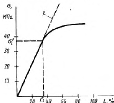
Диаграмма «напряжение — деформация»
