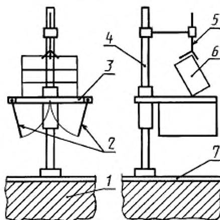
СХЕМА МАШИНЫ С РАСКРЫВАЮЩИМИСЯ СТВОРКАМИ ДЛЯ ИСПЫТАНИЙ ТАРЫ НА УДАР ПРИ СВОБОДНОМ ПАДЕНИИ
