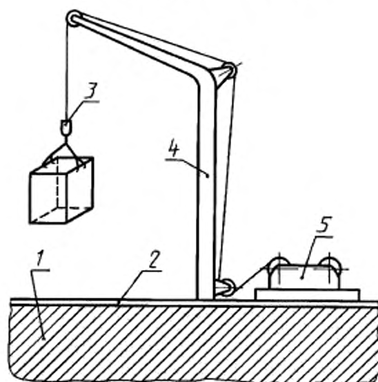
СХЕМА ПОДЪЕМНОГО УСТРОЙСТВА ДЛЯ ИСПЫТАНИЙ ТАРЫ НА УДАР ПРИ СВОБОДНОМ ПАДЕНИИ
