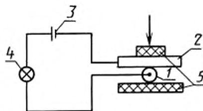
1 — образец; 2 — металлический брусок; 3 — источник питания; 4 — лампочка; 5 — пластинки
