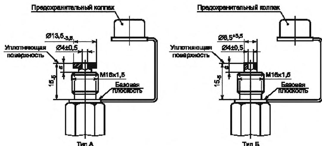
Рисунок А.2 — Присоединительные размеры клапанов контрольного вывода
