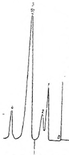
1—хлористый этил; 2—этиловый эфир; 3—бромистый этил; 4—этиловый спирт
