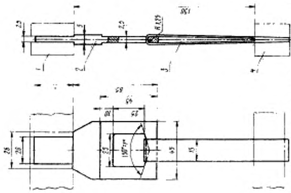
1—верхний зажим; 2—рамка; 3—образец; 4—нижний зажим Размер L — устанавливается в зависимости от размера зажима разрывной машины. Край выреза закруглить R 1,25 мм.
