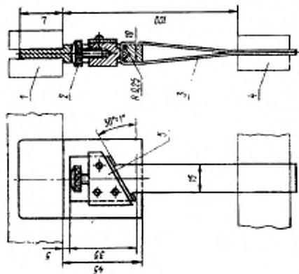
1—верхний зажим; 2—винт; 3—образец; 4—нижний зажим; 5—скользящий ползунок Размер L — устанавливается в зависимости от размера зажима разрывной машины.
