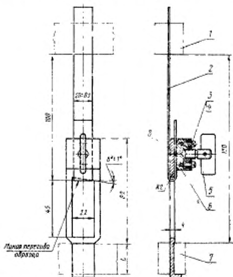
1 — верхний зажим; 2 — образец; 3 — винт специальный; 4 — пружина; 5 — винт; 6 — сухарь; 7 — нижний зажим; 8 — держатель.
