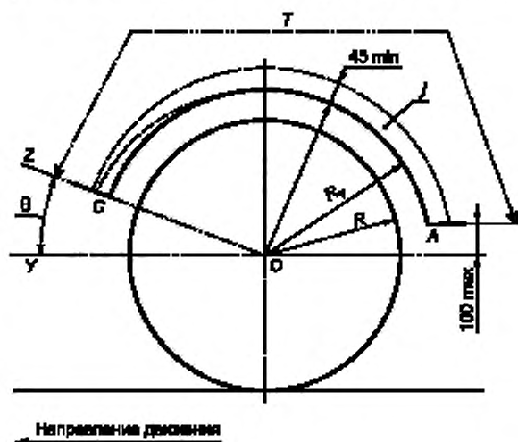
а) Расположение грязезащитного кожуха и наружной боковины
