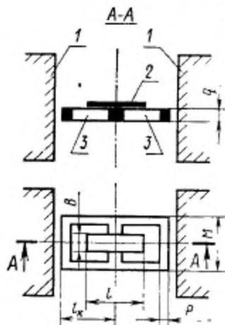
1—полюсные наконечники электромагнита; 2—образец; 3—катушки индукционного преобразователя
