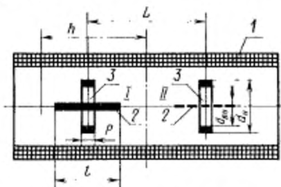
1—соленоид; 2—образец; 3—катушки индукционного преобразователя.
