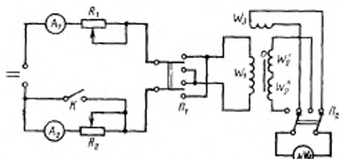
R_1, R_2 — регулировочные реостаты; A_1, A_2 — амперметры; K — ключ; P_1, P_2 — двухполюсные переключатели; W_2, W_2' — катушки индукционного преобразователя для измерения магнитного потока; W_2 — измерительная катушка; W_1 — обмотка намагничивающего устройства; \mu A — микрометр; O — образец.
