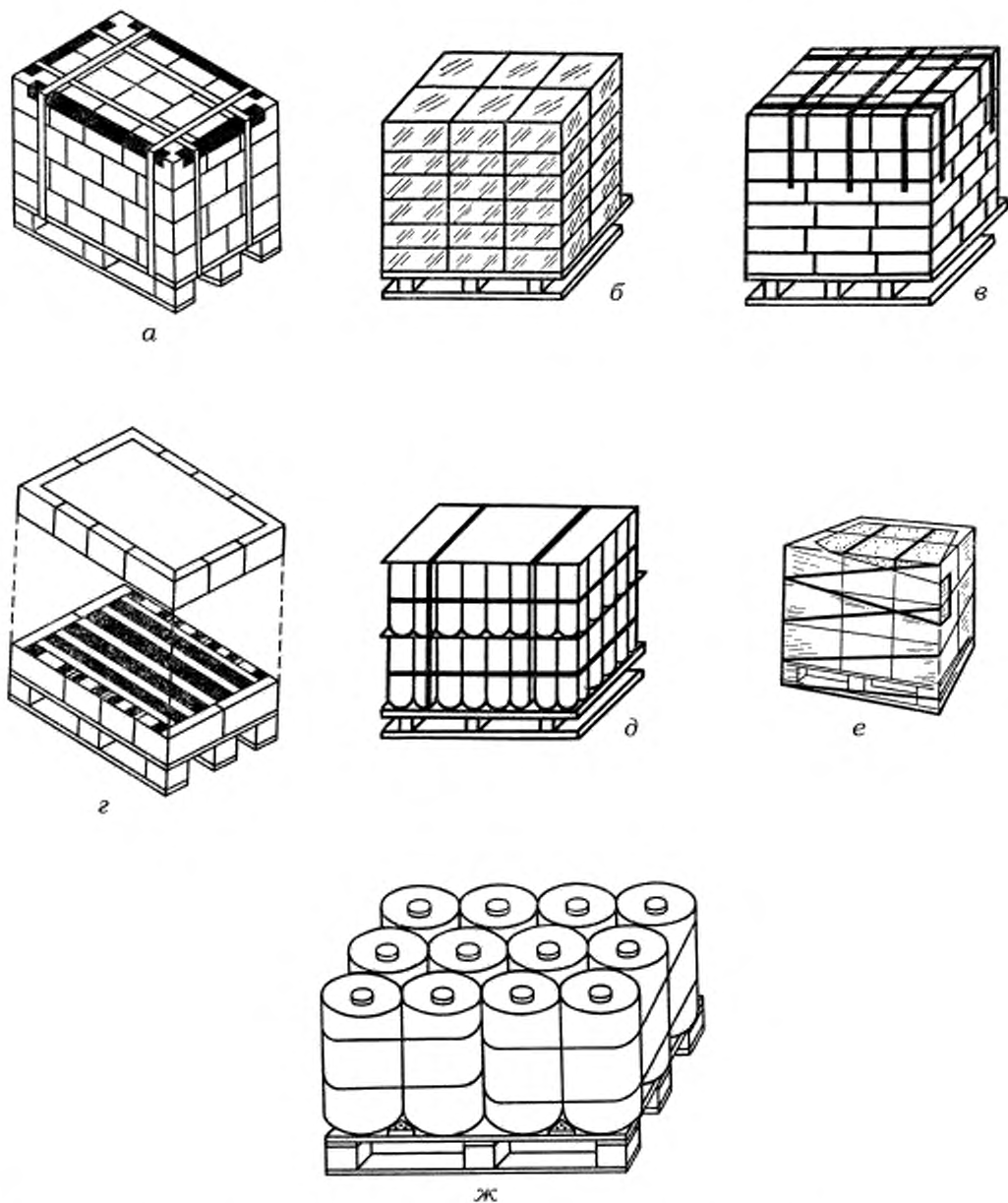
a — скрепление при помощи клея, ленты и уголков; б — скрепление пакетирующей пленкой; в — скрепление клейкой лентой; г — скрепление при помощи клея и kraft-бумаги; д — скрепление проволокой с применением картонных прокладок; е — скрепление при помощи растягивающейся пленки; ж — скрепление барабанов на поддоне
