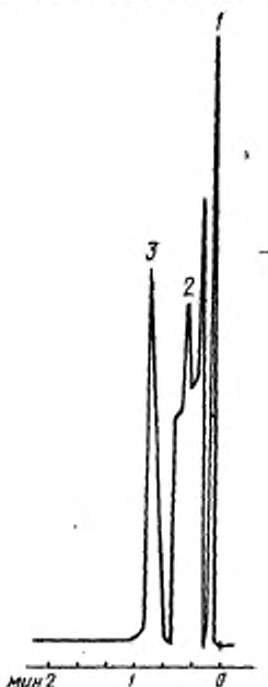
Типовая хроматограмма технического дифенила, полученная при 180°C
