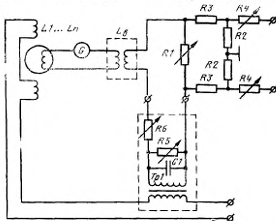
R_1 — регулировочное сопротивление; C_1 — емкость; Tr_1 — трансформатор; L_1 \dots L_n — набор регулировочных индуктивностей
