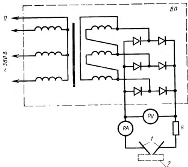
БП—блок питания; PV—вольтметр; РА—амперметр; R—резистор; I—электро- ды; 2—образец испытуемого материала
