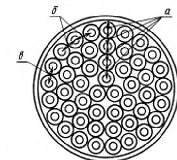
a, б, в — способы подключения, по которым изоляция жил подвергается испытанию.
