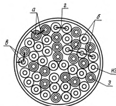
нэ — незэкранированная жила; э — отдельно экранированная жила; a, б, в, г, д, е, ж, з — способы подключения, по которым изоляция жил подвергается испытанию.
