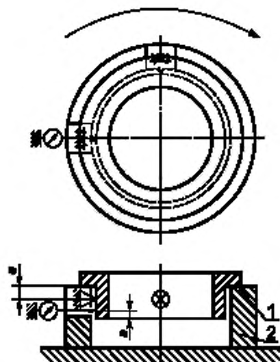
1 — опорный торец упорного борта; 2 — кольцообразная цилиндрическая опора, а — предел зоны измерения (таблица 57)
