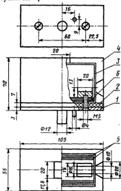
1—стальное основание камеры с фиксаторами; 2—асбоцементная плита; 3—стальная коробка; 4—теплоизоляция; 5—механизм; 6—электронагреватель
