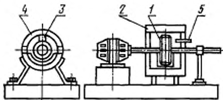
1—диск с испытуемой лентой; 2—камера с нагревательными; 3—защелка; 4—светлая контрольная лента; 5—термометр
