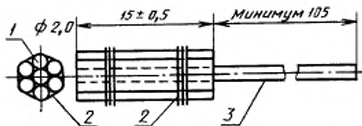
1 — сгруппированные провода диаметром 2,0 мм; 2 — медная проволока диаметром 0,35 мм; 3 — центральный провод (проволока)
