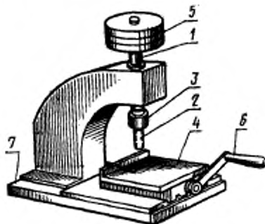
1—подвижной стержень; 2—плита с площадью поперечного сечения 1 см 2 ; 3—крепящая гайка; 4—плита передвижная; 5—грузы; 6—ручка для передвижения плиты; 7—направляющие салазки
