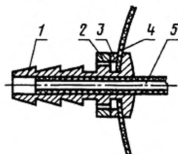
Схема крепления штуцера к СИЗ ОД
