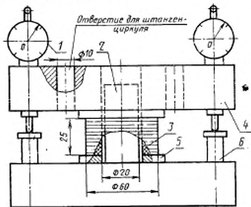
1—индикатор часового типа, 2—стержень для центрирования шайб; 3—набор шайб испытуемого электроизоляционного картона; 4—брусочки стальные; 5—шайба стальная; 6—штифты упорные стальные.
