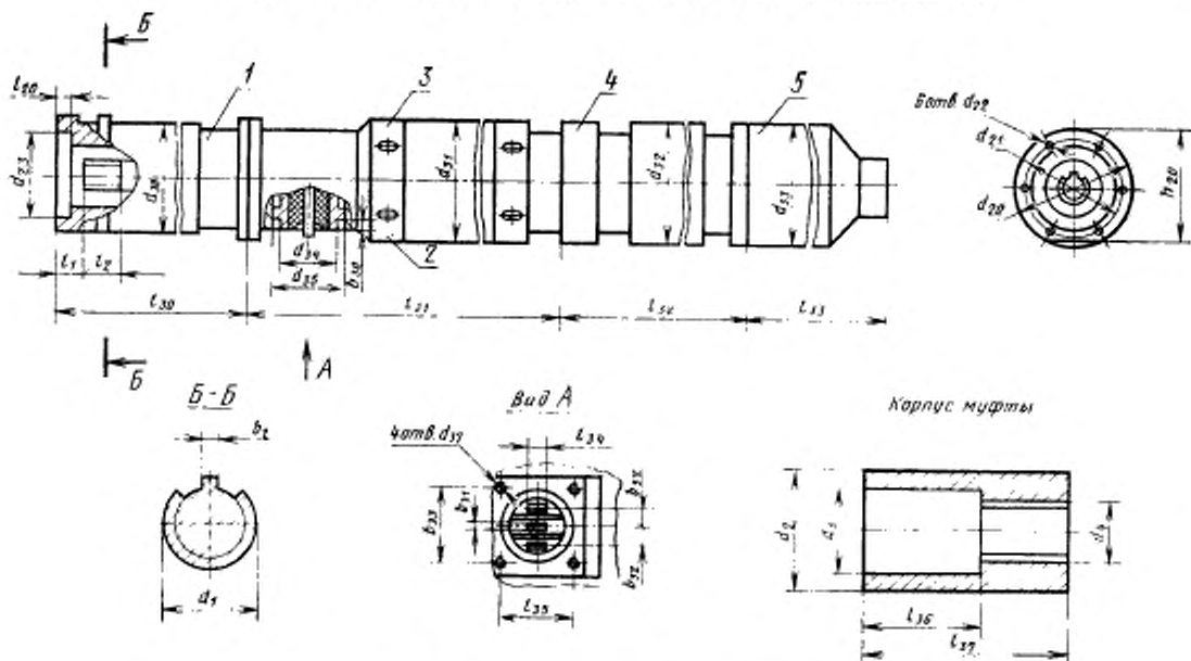
1—прожектор; 2—электродвигатель; 3—верхняя секция; 4—нижняя секция; 5—компенсатор
