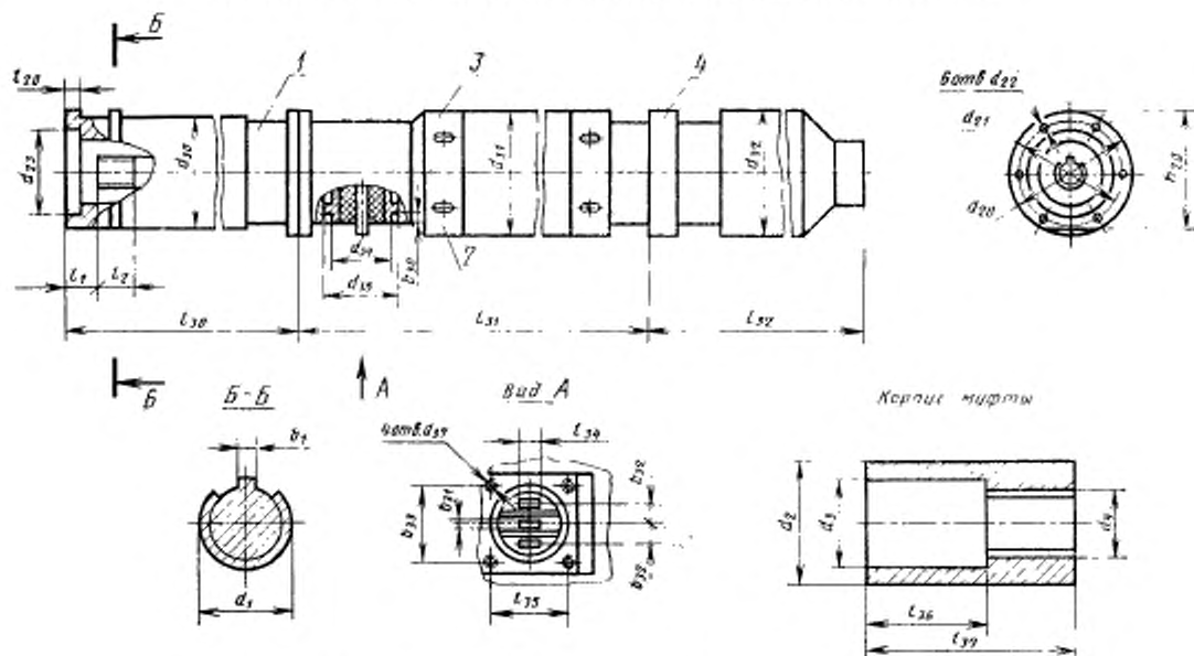
1—прожектор, 2—электродвигатель; 3—верхняя секция; 4—нижняя секция
