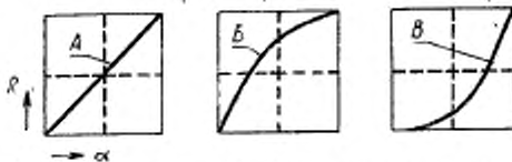
R — сопротивление; \alpha — рабочий угол поворота подвижной системы резистора; А — линейная зависимость; Б — нелинейная обратнологарифмическая зависимость; В — нелинейная логарифмическая зависимость.
