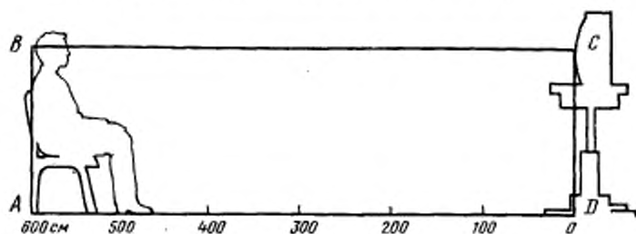
Схема расположения испытуателя и прибора типа ПОЗД-2
