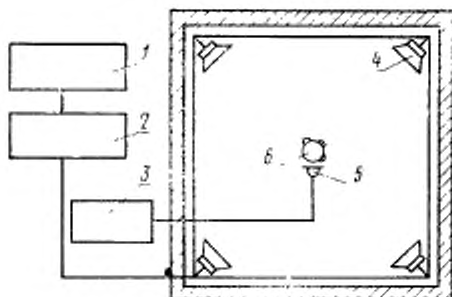
Принципиальная схема размещения измерительной аппаратуры
