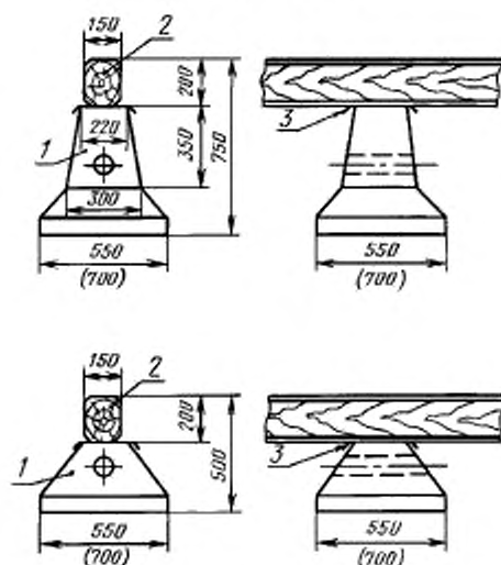
Опоры фундамента
