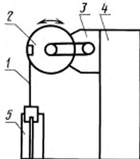
1 — испытуемый образец; 2 — сменные цилиндры; 3 — механизм вращения; 4 — стойка; 5 — натяжное устройство
