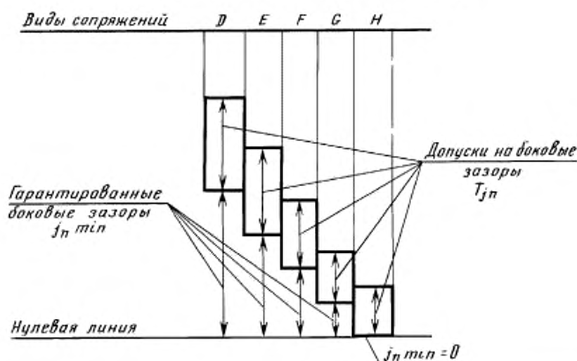
Виды сопряжений и гарантированные боковые зазоры
