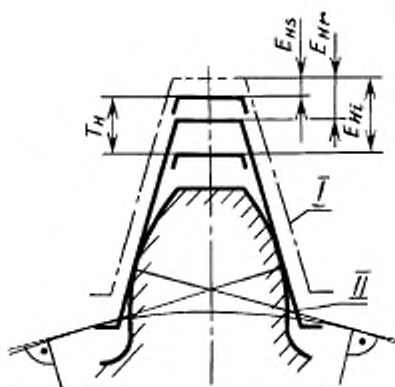
I — номинальное положение исходного контура, II — действительное положение исходного контура
