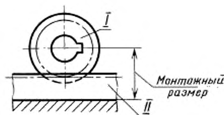
I — зубчатое колесо; II — рейка
