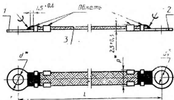
Перемишка типа Б
