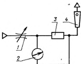
1—дрозель; 2—манометр; 3—аппарат; 4—ротаметр.
