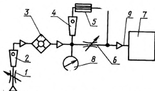
1—дрозель; 2—ротаметр; 3—испаритель анестетиков; 4—ротаметр; 5—устройство для измерения концентрации паров наркотизирующих веществ; 6—дрозель; 7—вытяжной шкаф; 8—насос; 9—газотводящий шланг.
