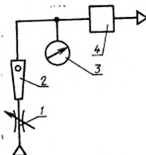
1—дрозель; 2—ротаметр; 3—манометр; 4—аппарат (предохранительный клапан).
