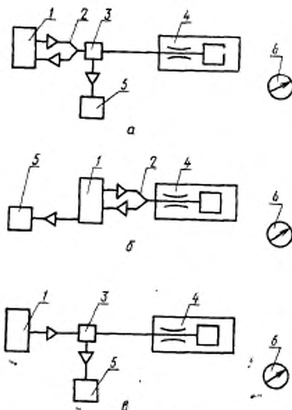
1—аппарат ИВЛ; 2—тройник нациента; 3—неревверсивный клапан; 4—модель легких; 5—спирометр; 6—секундомер.
