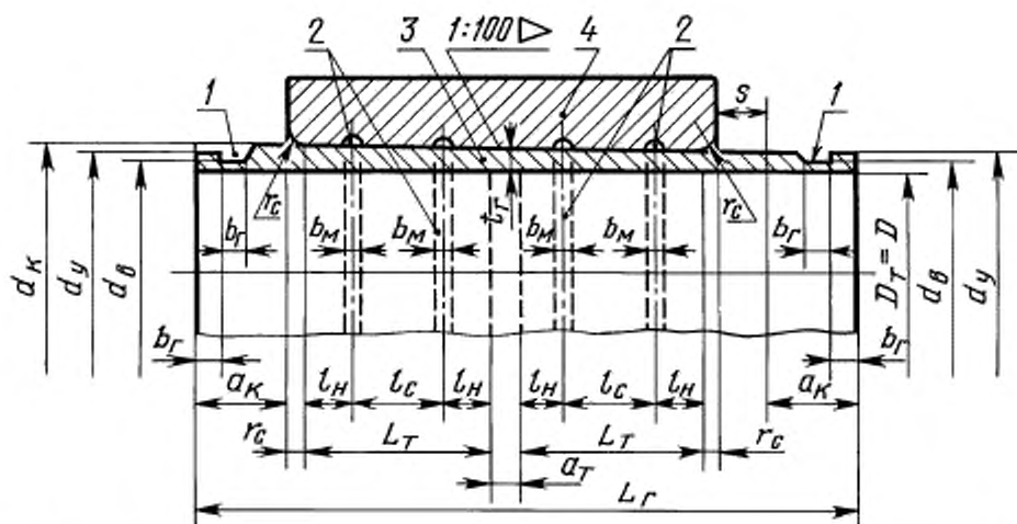
Исполнение 2 (при D > 140 мм)
