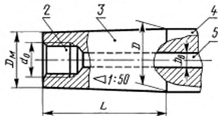
Исполнение 2 (для соединения типа III)
