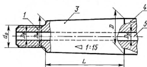
Исполнение 1 (для соединений типов I и II)
