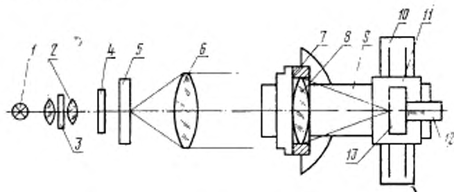
1 — источник света; 2 — конденсор; 3 — светофильтр; 4 — матовое стекло; 5 — тест-объект; 6 — объектив коллиматора; 7 — опорный торец объективодержателя; 8 — испытуемый объектив; 9 — поворотный рычаг с продольными направляющими; 10 — поперечные направляющие; 11 — каретка, перемещаемая по поперечным направляющим; 12 — микрометрический механизм продольного перемещения; 13 — приемник изображения
