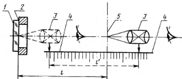
1—стеклянная пластина; 2—опорный торец объективодержателя; 3—микроскоп; 4—отсчетная шкала механизма продольного перемещения микроскопа; 5—положение наилучшей плоскости изображения объектива; l —размер рабочего отрезка
