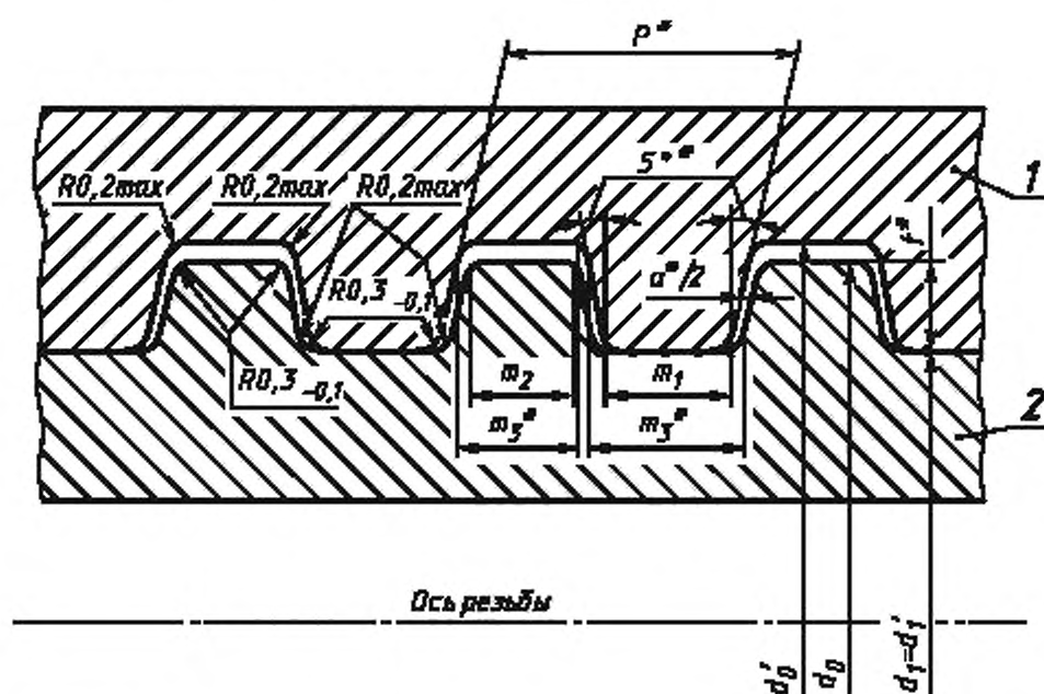
Черт. 1
