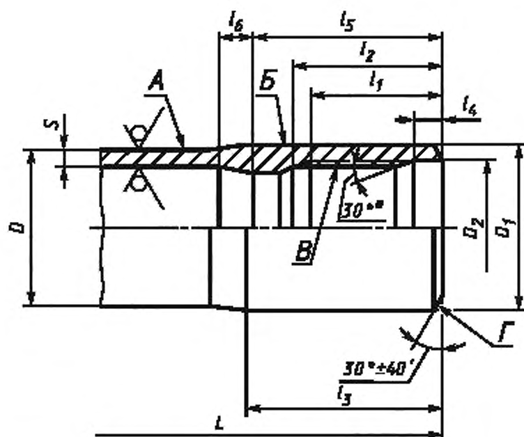
Черт. 1
