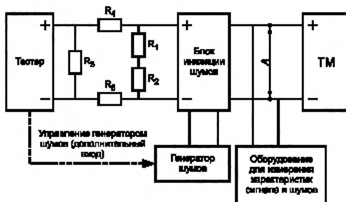
Рисунок 8 — Схема тестирования помехоустойчивости ТМ
