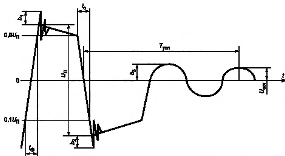
Рисунок 4 — Характеристики выходного сигнала ТМ
