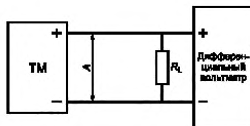
Рисунок 3 — Схема измерения выходного шума ТМ
