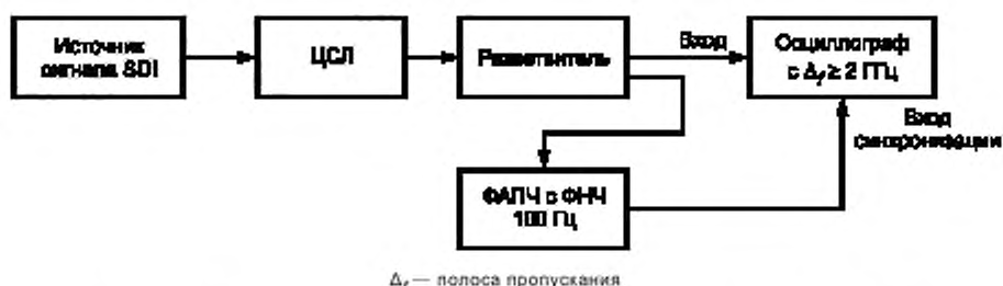
Рисунок 9 — Схема измерения высокочастотного фазового дрожания цифрового сигнала
