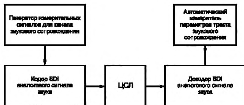
Рисунок 12 — Схема измерения параметров канала звукового сопровождения
