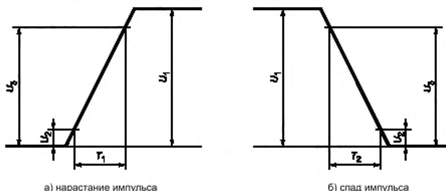
Рисунок 4 — Диаграммы, поясняющие измерение времени нарастания и спада импульса
