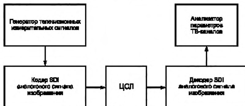
Рисунок 11 — Схема измерения параметров канала изображения
