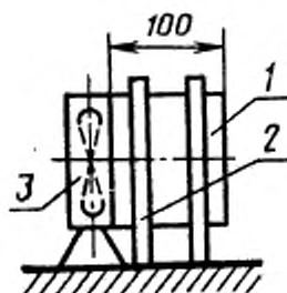
1—цилиндр; 2—стойка; 3—вентилятор
