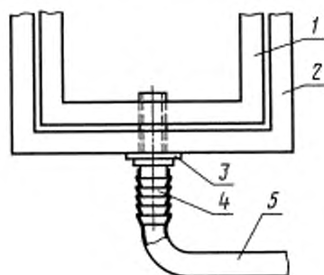
Схема крепления штуцера к рамке
