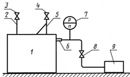
1 — резервуар; 2 — всасывающий трубопровод; 3, 4 — запорные краны; 5 — нагнетающий трубопровод; 6 — уравниватель; 7 — манометр; 8 — пус- ковой кран; 9 — компрессор
