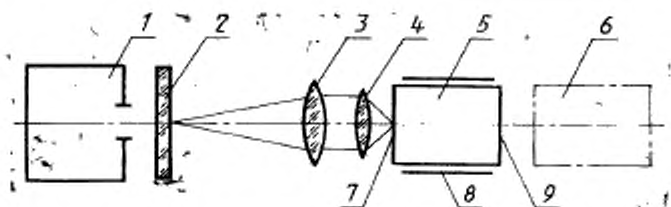
1—осветитель; 2—сетка; 3—коллимационный объектив; 4—проекционный объектив; 5—ЭОП; 6—источник; 7—фотокатод; 8—светонепроницаемая камера; 9—экран
