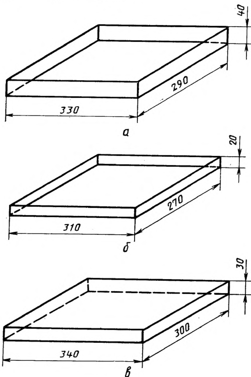
а—поддон; б—прижимная рамка; в—крышка
