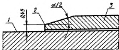
1 — поверхность стебля; 2 — измерительная кромка; 3 — барабан
