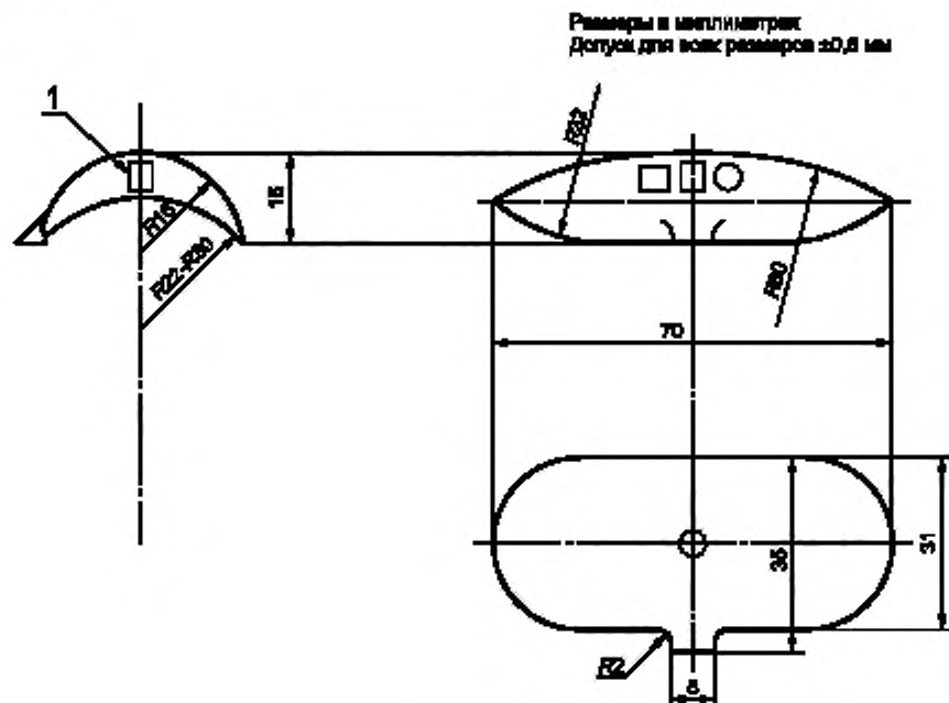
1 — акселерометр
