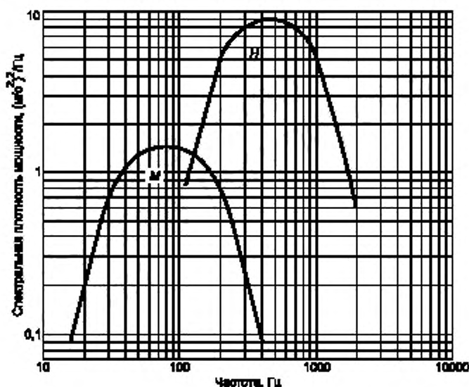
Рисунок 6 — Спектры двух сигналов вибрации (М и Н), измеряемых на рукоятке
