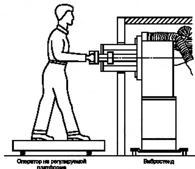
Рисунок 4 — Положение оператора в ходе испытаний
