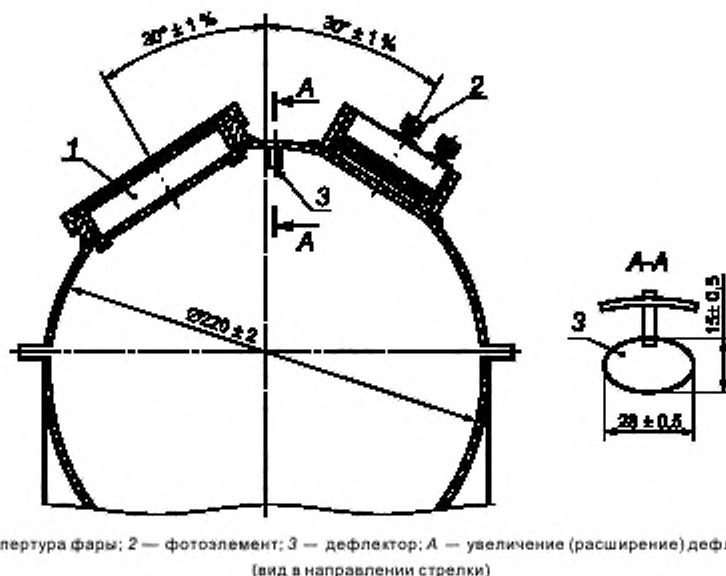
Рисунок А.1 — Схема светомерного шара
