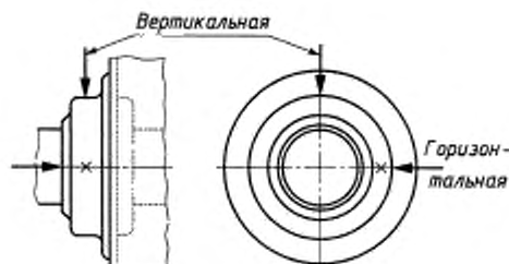
Рисунок 1б — Точки измерения на корпусе подшипника
