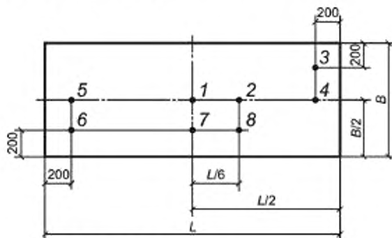
1, 2, 3, 4, 5, 6, 7, 8 — точки приложения нагрузки
