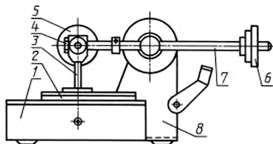
1 — корпус; 2 — платформа; 3 — контактная головка; 4 — муфта; 5 — груз; 6 — противовес; 7 — двуплечный рычаг; 8 — стойка
