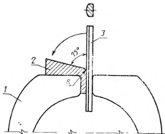
1—тиски; 2—накладка; 3—образец
