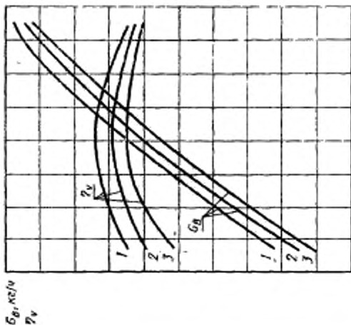
1, 2, 3—при различных P —const Черт. 13
