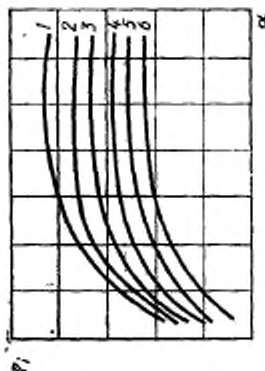
Зависимости индикаторного КПД от коэффициента избытка воздуха
