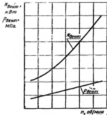
Черт. 20
