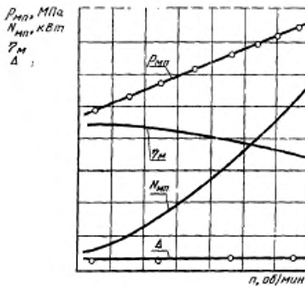
Черт. 7
