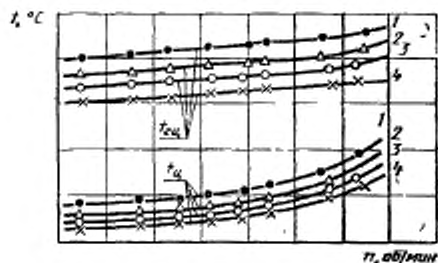
Черт. 18
