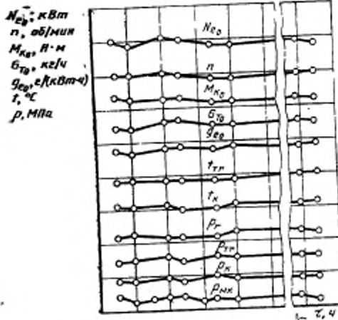
Черт. 26
