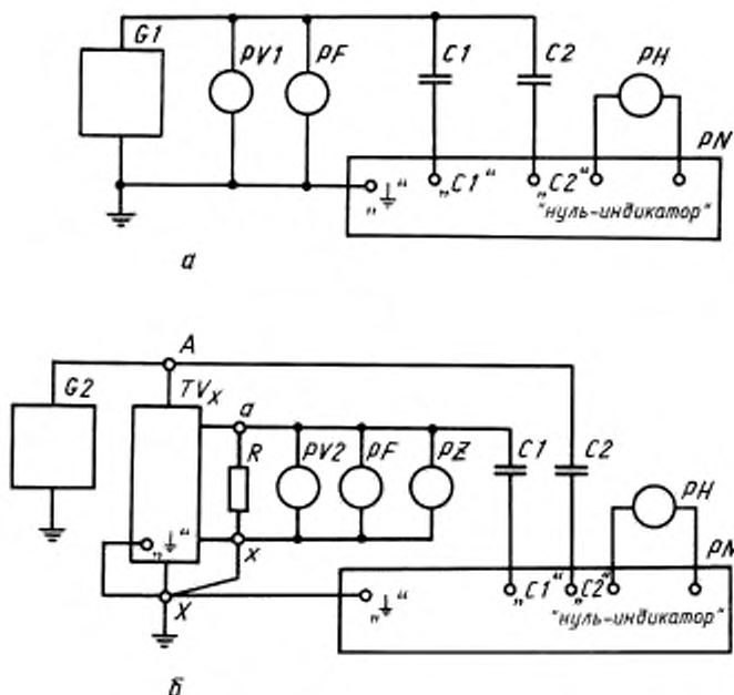
Схема проверки однофазного трансформатора методом компарирования токов
