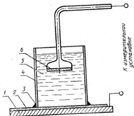
1 — металлический образец; 2 — испытываемое покрытие; 3 — уплотнительная замазка; 4 — толстый стеклянный цилиндр; 5 — раствор хлористого натрия; 6 — платиновый электрод.
