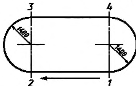
Рисунок А.1 — Испытательный полигон
