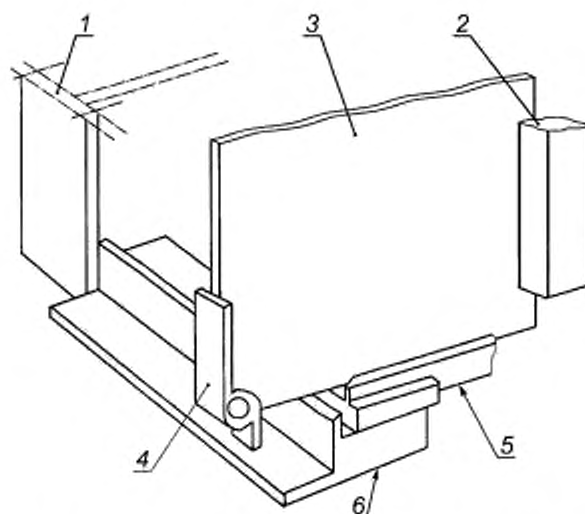
1 — типовый монтажный фланец блочного каркаса; 2 — соединитель; 3 — печатная плата; 4 — рукоятка инжектора-экстрактора, установленная на печатной плате; 5 — типовая направляющая; 6 — типовая горизонтальная деталь
