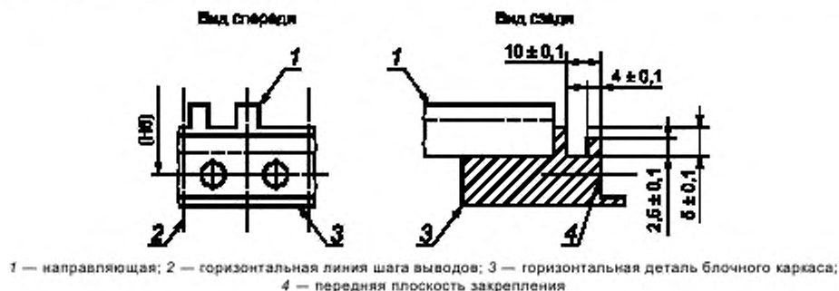
Рисунок 5 — Сопрягающиеся размеры блочного каркаса для печатной платы с установленными рукоятками инжектора-экстрактора типа В
