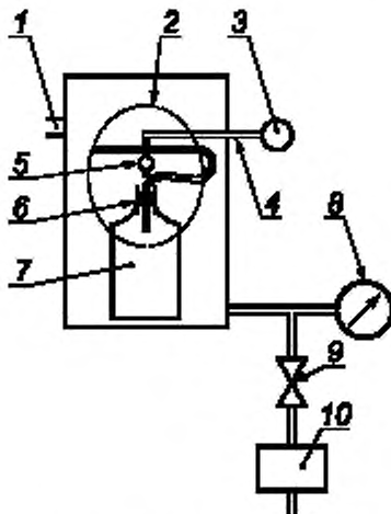
1 — соединение изолирующего устройства с рабочим трубопроводом; 2 — смотровое окно; 3 — резиновая груша с пипеткой; 4 — резиновая трубка; 5 — трубка Парджо; 6 — резиновая пробка; 7 — стеклянный сосуд; 8 — манометр; 9 — изолирующий вентиль; 10 — источник давления или вакуума
