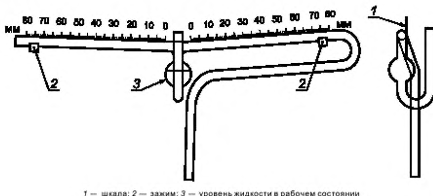
Рисунок F.4 — Трубка Парджо (тип А)
