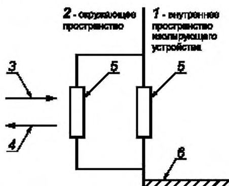
Рисунок D.3 — Передаточное устройство типа В1
