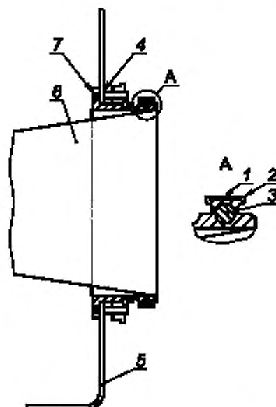
1 — узел крепления перчатки (хомут, бугель); 2 — сдавливающая манжета; 3 — уплотнительное кольцо; 4 — уплотнение; 5 — корпус изолирующего устройства (внутренняя сторона); 6 — перчатка; 7 — перчаточный порт
