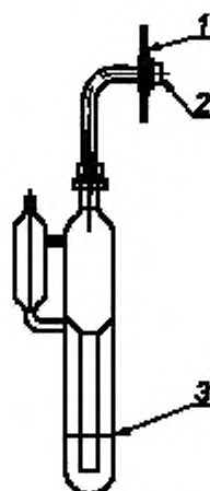
1 — панель; 2 — направление от НЕРА фильтра; 3 — уровень масла
