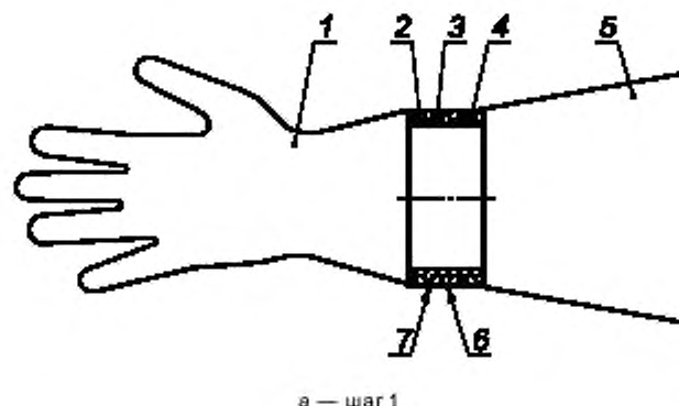
1 — перчатка; 2 — уплотнительное кольцо перчатки; 3 — кольцо манжеты; 4 — уплотнительное кольцо рукава; 5 — рукав; 6 — кромка рукава; 7 — кромка перчатки
