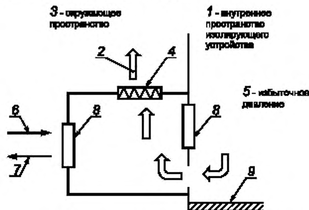
Рисунок D.5 — Передаточное устройство типа С1
