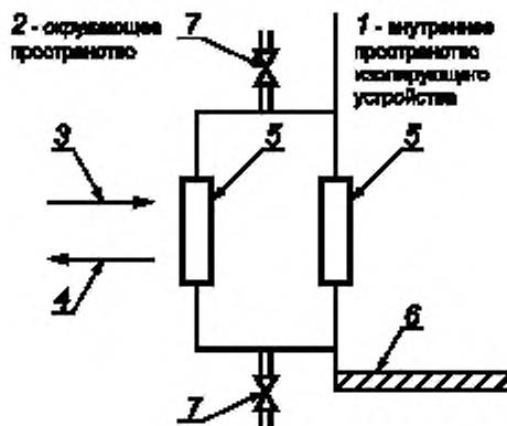
Рисунок D.4 — Передаточное устройство типа В2
