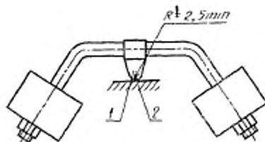
1 — сфера; 2 — образец
