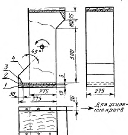
1 — барашковая плита; 2 — сталь; 3 — резина; 4 — гладкий пластмассовый лист
