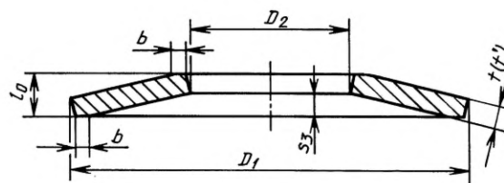
Пружина типа 2
